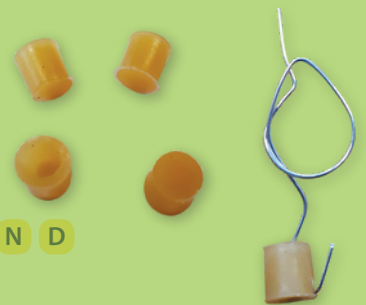
Phéromone d'agrégation
